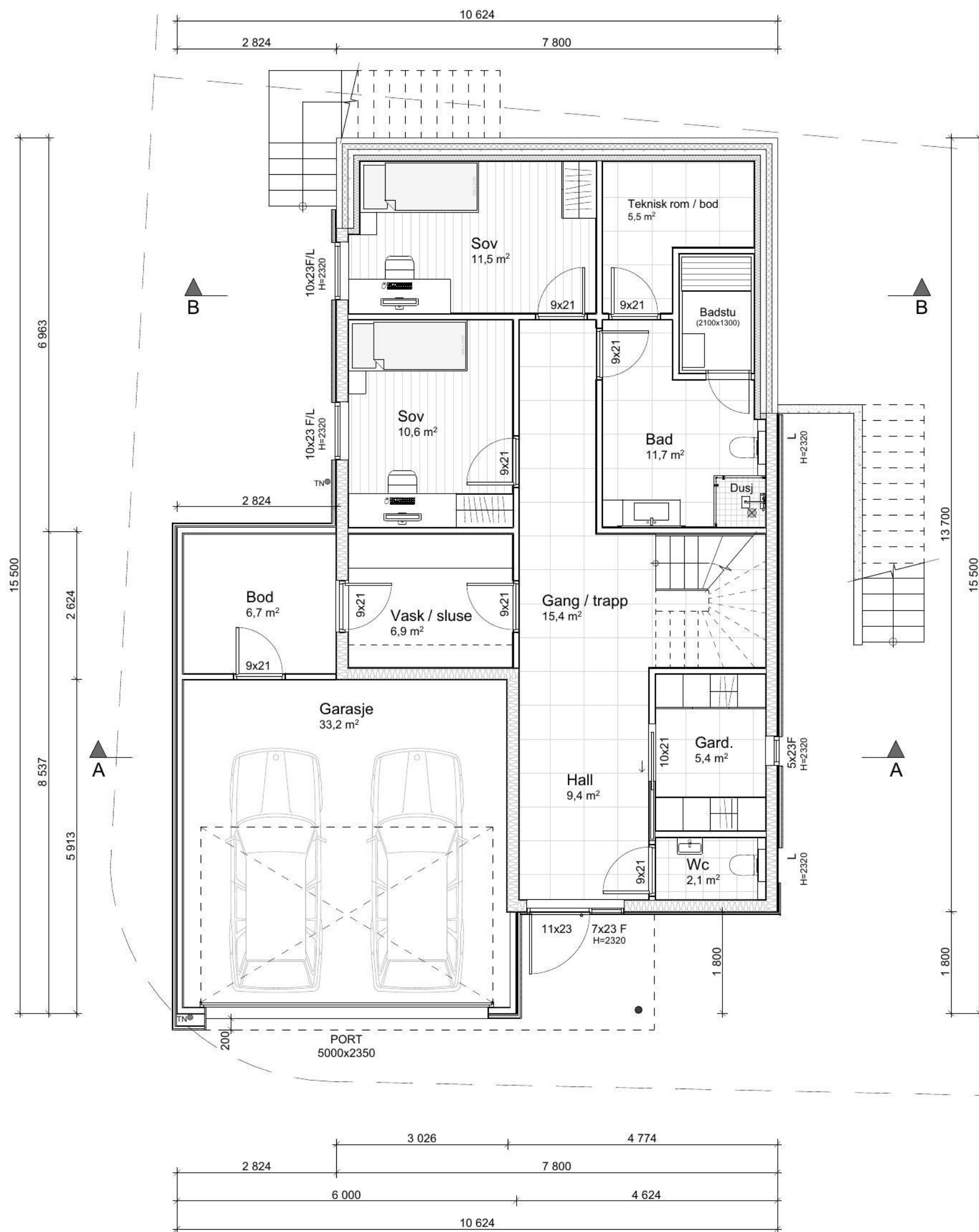
Plan 1.etasje BRA bolig B (inkl. garasje) 125,2 m²
